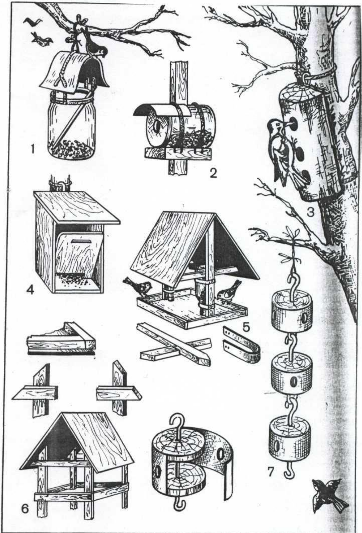
Кормушки для птиц: 1, 2 — из стеклянных банок; 3 — из полена для дятла; 4, 5, 6 — домики; 7 — фонарь.
